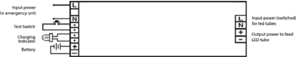
Aansluitschema
